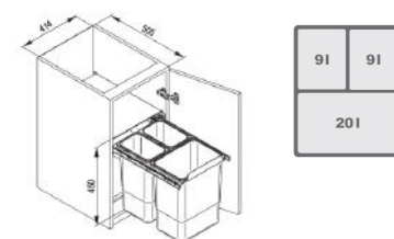
JC606 45 WYSOKI DO SZAFKI 50 CM
