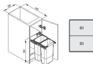
ALADIN 2 DO SZAFKI 40 CM
